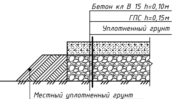
Конструкция бетонное покрытие проезжей части (П-3)
