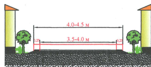
Андолавий қўндаланг кесимлар
