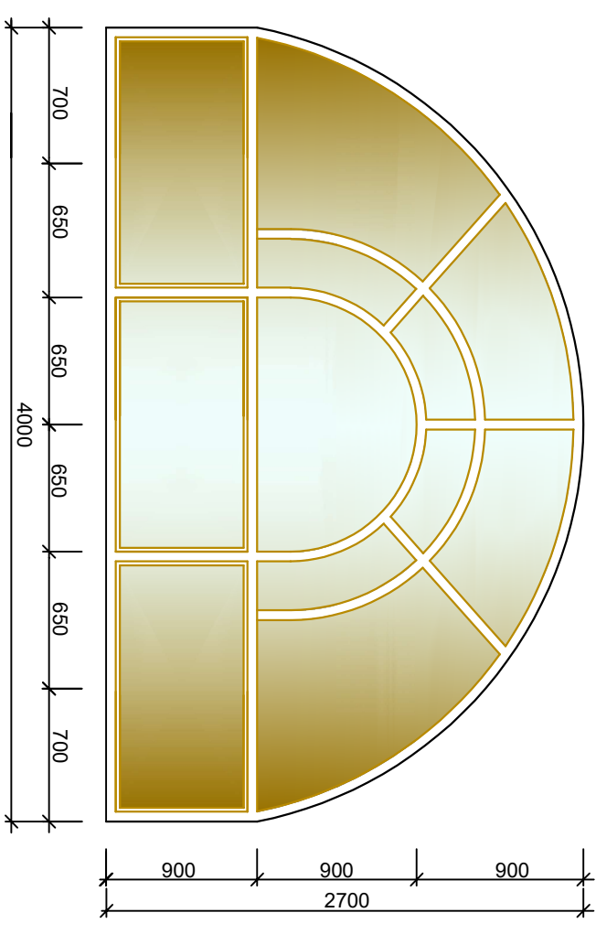
Витраж В-1(из алюминиевого профиля типа "АКФА" с остеклением) 2-шт
