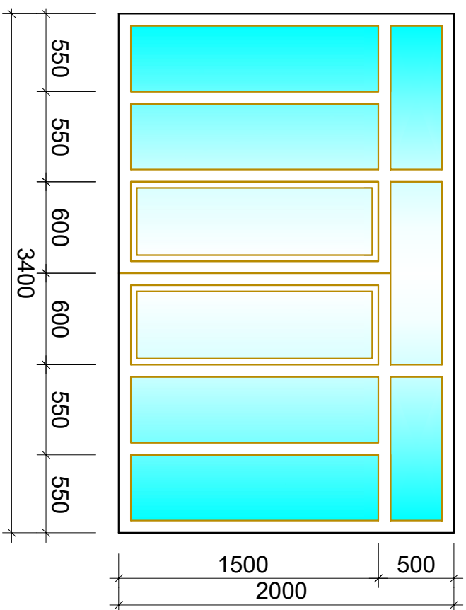
Витраж В-13(из алюминиевого профиля типа "АКФА" с остеклением) 1-шт
