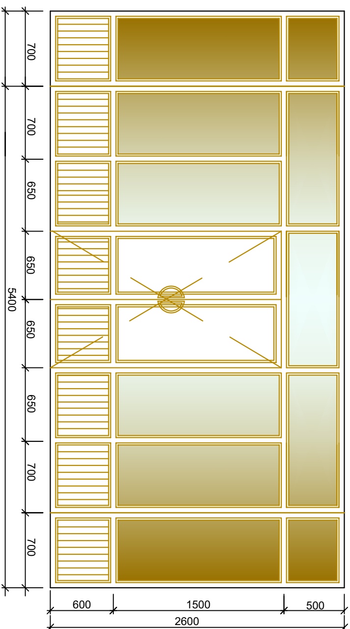
Витраж В-4(из алюминиевого профиля типа "АКФА" с остеклением) 2-шт
