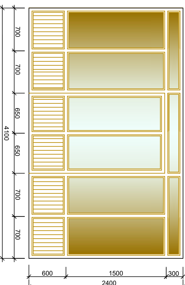
Витраж В-7(из алюминиевого профиля типа "АКФА" с остеклением) 1-шт
