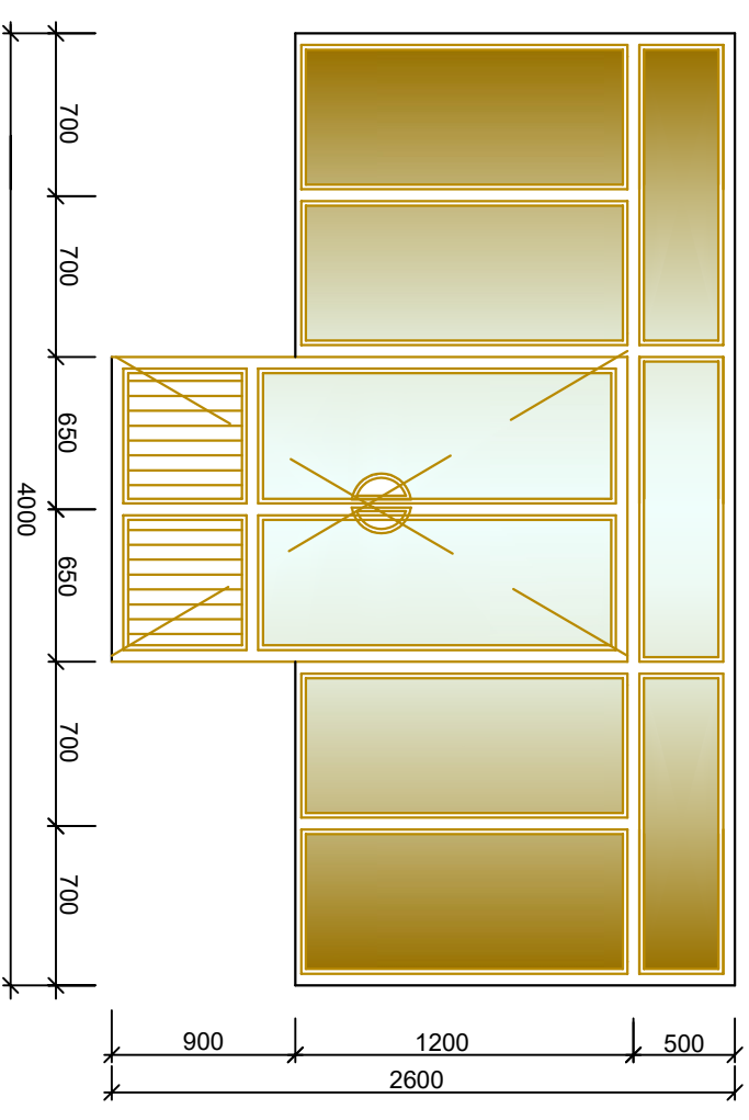
Витраж В-12(из алюминиевого профиля типа "АКФА" с остеклением) 1-шт
