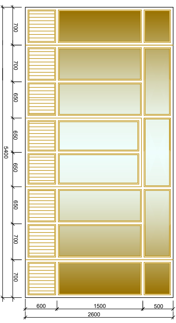
Витраж В-5(из алюминиевого профиля типа "АКФА" с остеклением) 1-шт
