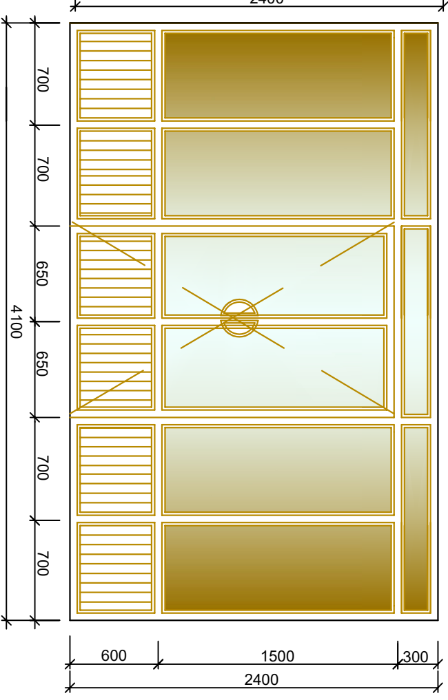
Витраж В-8(из алюминиевого профиля типа "АКФА" с остеклением) 1-шт
