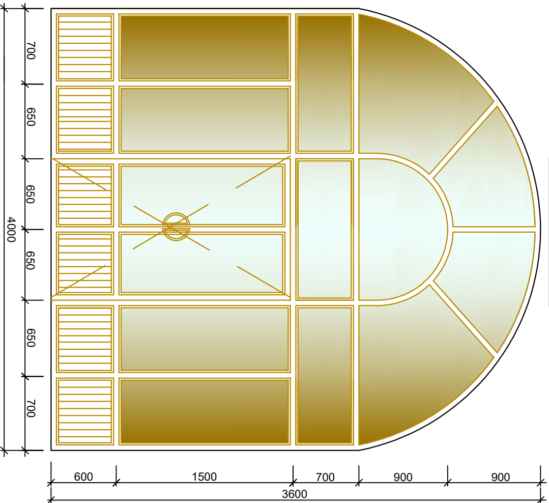
Витраж В-13(из алюминиевого профиля типа "АКФА" с остеклением) 1-шт
