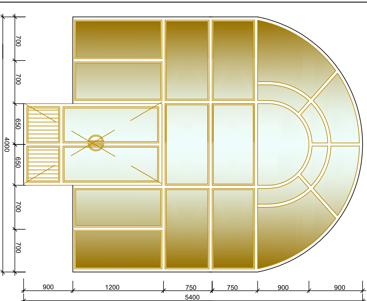
Витраж В-6(из алюминиевого профиля типа "АКФА" с остеклением) 1-шт
