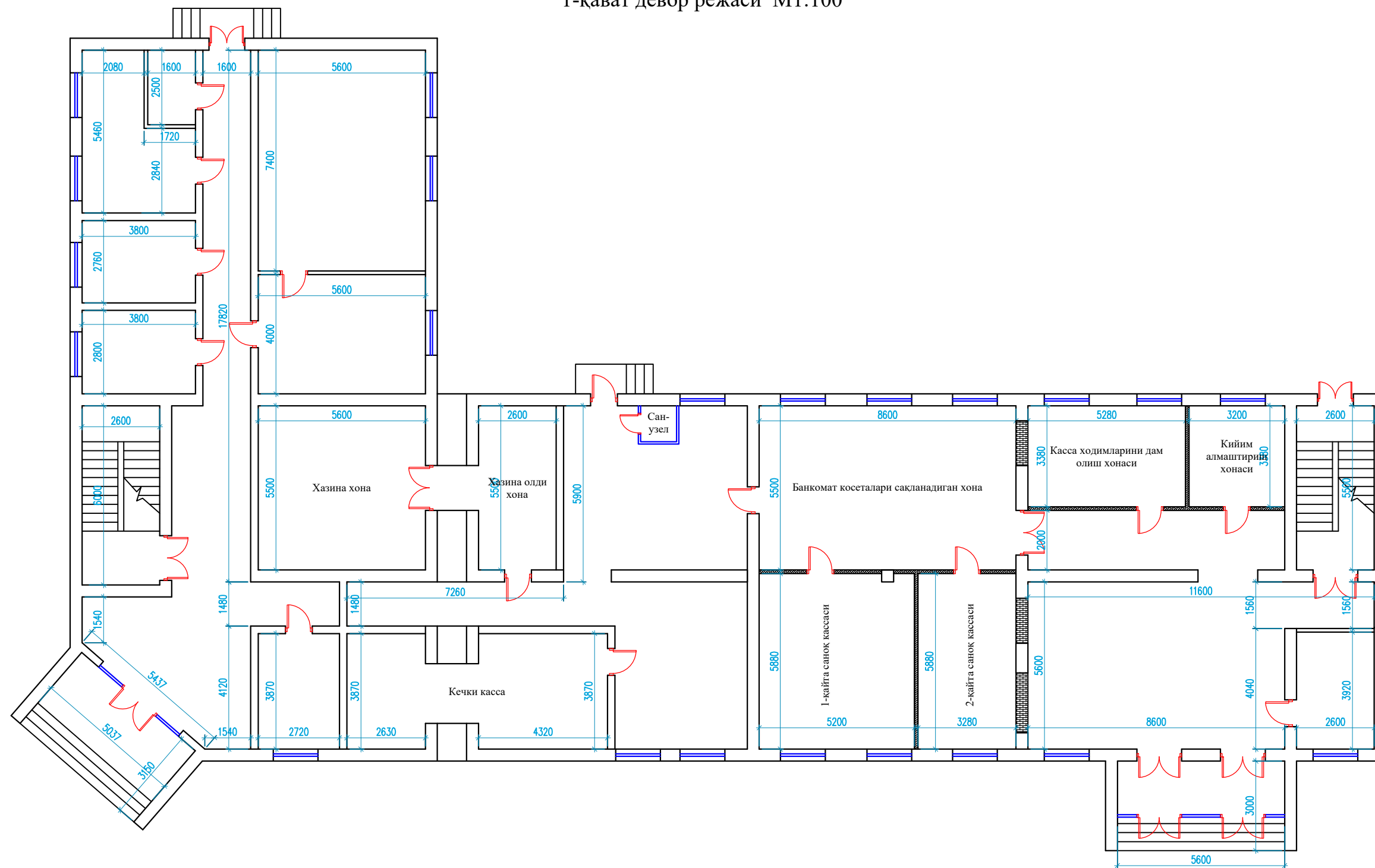
1-қават девор режаси М1:100
